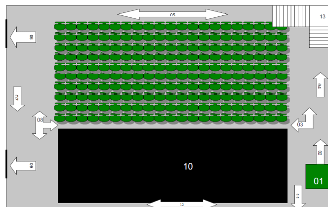
TEATRO SESC PATATIVA DO ASSARÉ (lay-out Piso Térreo – formato palco italiano)
